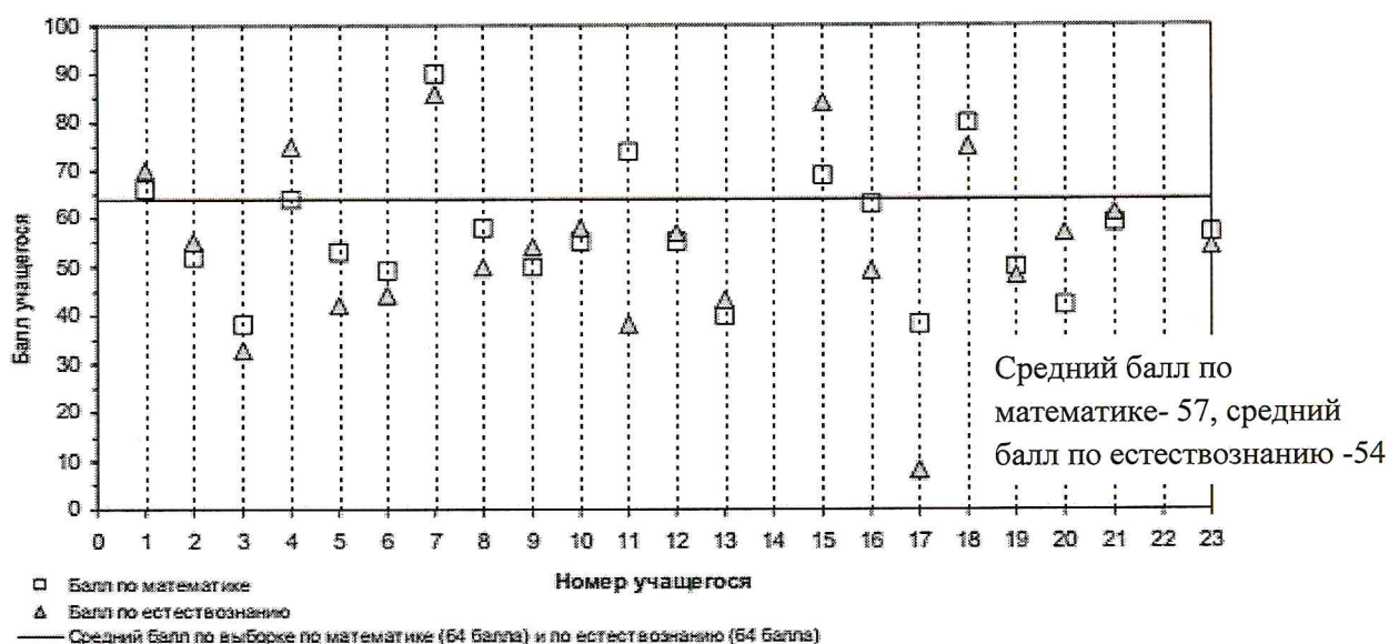
Рис 1. Результаты выполнения тестов международного исследования TIMSS-2015 по математике и естествознанию учащимися данного класса
